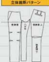
「ダブルアクション」パンツの立体裁断パターン
